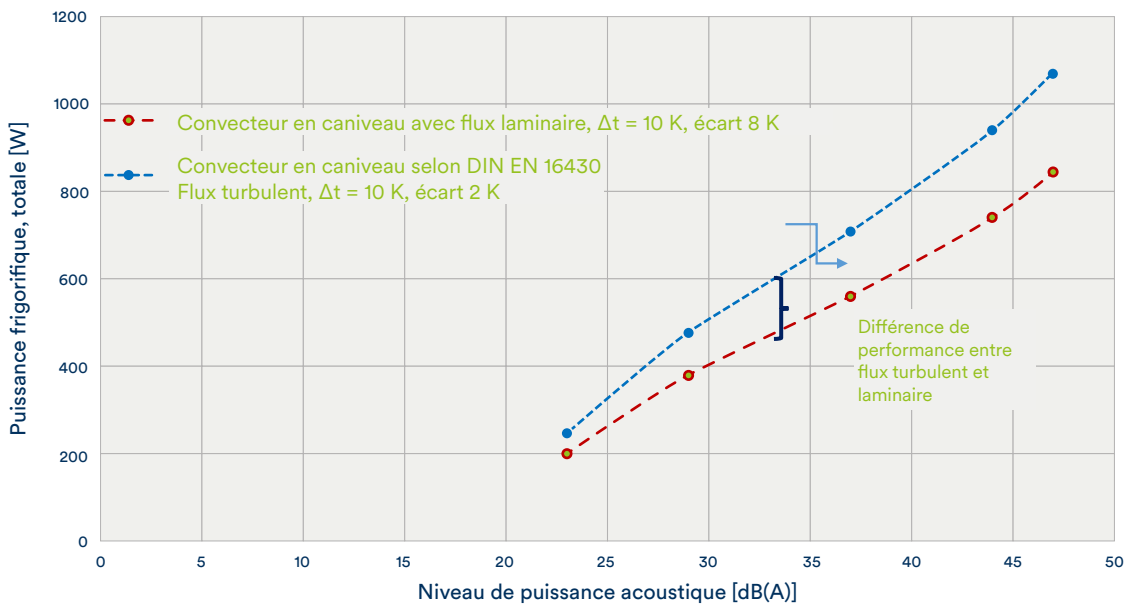
Comparaison des performances - Influence d'un flux laminaire
